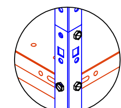
ENCAIXE DA COLUNA
