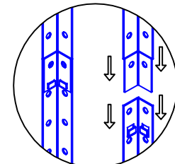
ENCAIXE DA COLUNA
